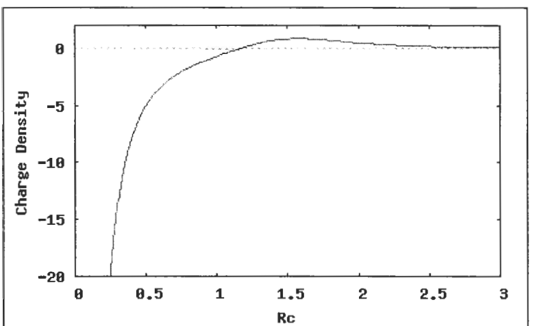
Fig. 6a-d. Generalized Kerr-Newman, q=2 , a=1 , \alpha=1 , \theta=\pi/2
